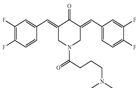
3,5-Bis((E)-3,4-difluorobenzylidene)-1-(4-(dimethylamino)butanoyl)piperidin-4-one (JC068)
