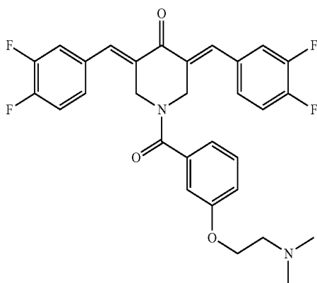
3,5-Bis((E)-3,4-difluorobenzylidene)-1-(3-(2-(dimethylamino)ethoxy)benzoyl)piperidin-4-one (JC085)
