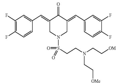
1-((2-(Bis(2-methoxyethyl)amino)ethyl)sulfonyl)-3,5-bis((E)-3,4-difluorobenzylidene)piperidin-4-one (JC107)
