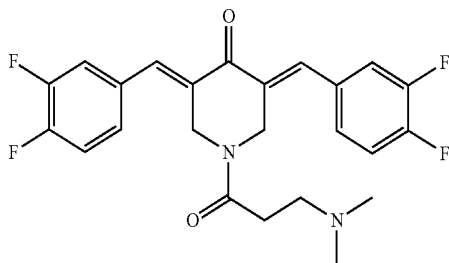
3,5-Bis((E)-3,4-difluorobenzylidene)-1-(3-(dimethylamino)propanoyl)piperidin-4-one (JC026)
