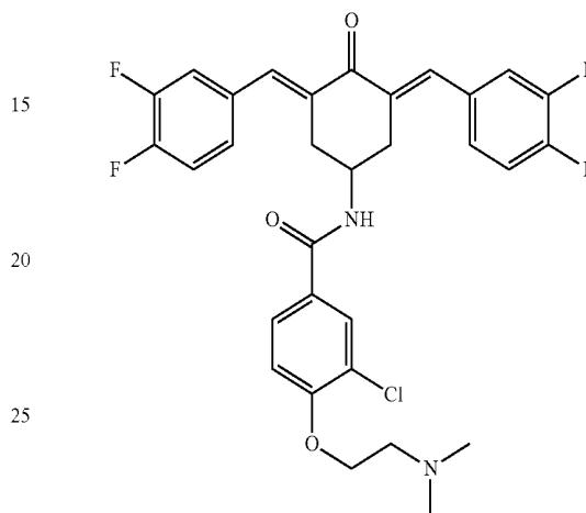
N-(3,5-Bis((E)-3,4-difluorobenzylidene)-4-oxocyclohexyl)-3-fluoro-4-(2-(dimethylamino)ethoxy)benzamide (JC117)
