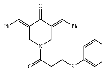
3,5-Di((E)-benzylidene)-1-(3-(phenylthio)propanoyl)piperidin-4-one (JC012)
