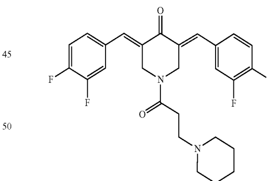
3,5-Bis((E)-3,4-difluorobenzylidene)-1-(3-(piperidin-1-yl)propanoyl)piperidin-4-one (JC048)
