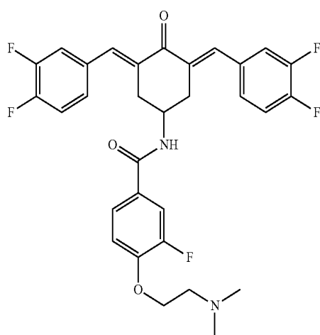
N-(3,5-Bis((E)-3,4-difluorobenzylidene)-4-oxocyclohexyl)-3-chloro-4-(2-(dimethylamino)ethoxy)benzamide (JC118)
