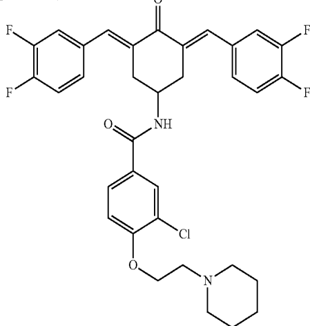
N-(3,5-Bis(E)-3,4-difluorobenzylidene)-4-oxocyclohexyl-3-chloro-4-(2-(piperidin-1-yl)ethoxy)Benzamide (JC113)
