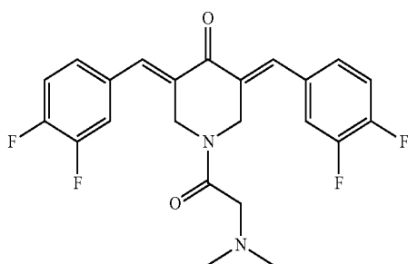
3,5-Bis((E)-3,4-difluorobenzylidene)-1-(dimethylglycyl)piperidin-4-one (JC061)
