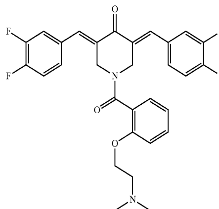
3,5-Bis((E)-3,4-difluorobenzylidene)-1-(2-(2-(dimethylamino)ethoxy)benzoyl)piperidin-4-one (JC086)
