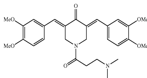
3,5-Bis((E)-3,4-dimethoxybenzylidene)-1-(3-(dimethylamino)propanoyl)piperidin-4-one (JC029)
