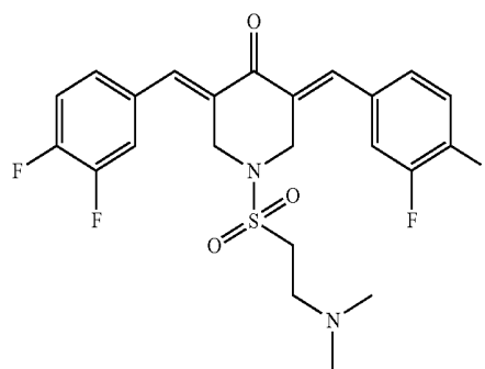
3,5-Bis((E)-3,4-difluorobenzylidene)-1-((2-(dimethylamino)ethyl)sulfonyl)piperidin-4-one (JC060)
