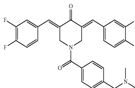
3,5-Bis((E)-3,4-difluorobenzylidene)-1-(4-((dimethylamino)methyl)benzoyl)piperidin-4-one (JC087)
