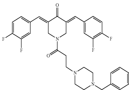
1-(3-(4-Benzylpiperazin-1-yl)propanoyl)-3,5-bis((E)-3,4-difluorobenzylidene)piperidin-4-one (JC051)
