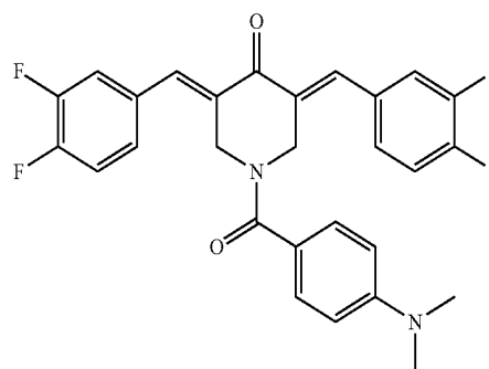
3,5-Bis((E)-3,4-difluorobenzylidene)-1-(4-(dimethylamino)benzoyl)piperidin-4-one (JC074)
