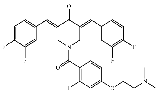
3,5-Bis((E)-3,4-difluorobenzylidene)-1-(4-(2-(dimethylamino)ethoxy)-2-fluorobenzoyl)piperidin-4-one (JC084)
