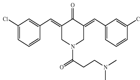
3,5-Bis((E)-3-chlorobenzylidene)-1-(3-(dimethylamino)propanoyl)piperidin-4-one (JC017)
