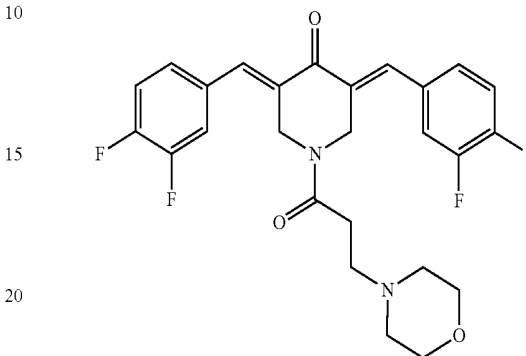
3,5-Bis((E)-3,4-difluorobenzylidene)-1-(3-morpholinopropanoyl)piperidin-4-one (JC047)
