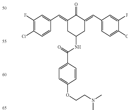
N-(3,5-Bis((E)-3,4-difluorobenzylidene)-4-oxocyclohexyl)-3-chloro-4-(2-(dimethylamino)ethoxy)benzamide (JC118)
