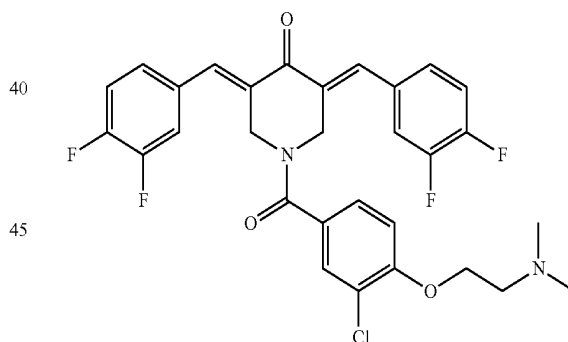
1-(3-Chloro-4-(2-(dimethylamino)ethoxy)benzoyl)-3,5-bis((E)-3,4-difluorobenzylidene)piperidin-4-one (JC083)
