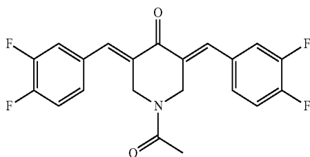
1-Acetyl-3,5-bis((E)-3,4-difluorobenzylidene)piperidin-4-one (JC106)
