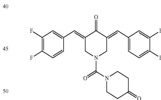
3,5-Bis((E)-3,4-difluorobenzylidene)-1-(4-oxopiperidine-1-carbonyl)piperidin-4-one (JC093)
