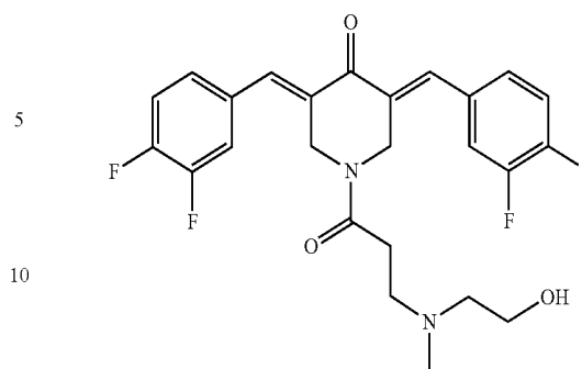
3,5-Bis((E)-3,4-difluorobenzylidene)-1-(3-((2-hydroxyethyl)(methyl)amino)propanoyl)piperidin-4-one (JC052)
